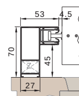
Führungsschiene ED53V
