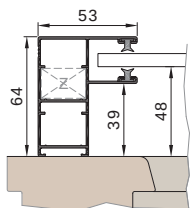
Führungsschiene KD53V
