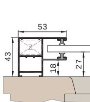
Führungsschiene KA53V
