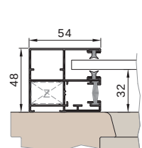
Führungsschiene KR54V
